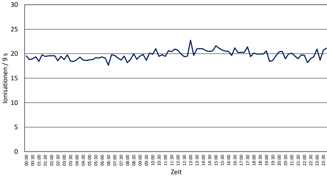
Anzahl Ionisationen
