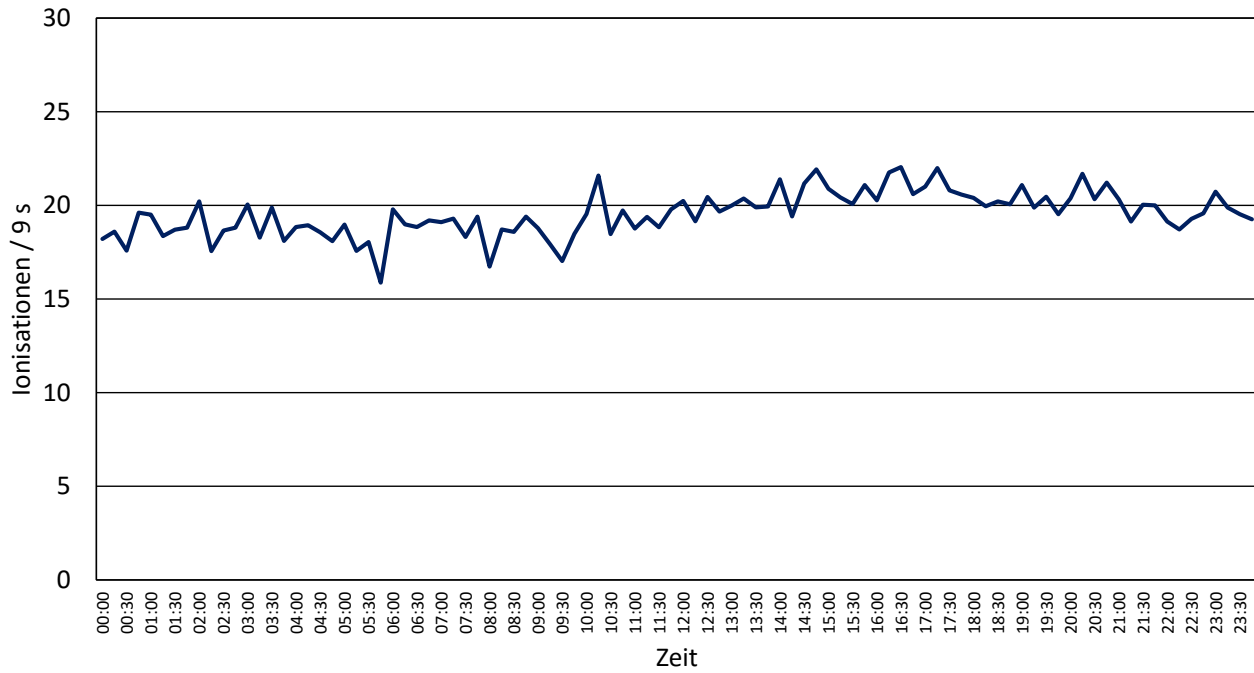
Anzahl Ionisationen
