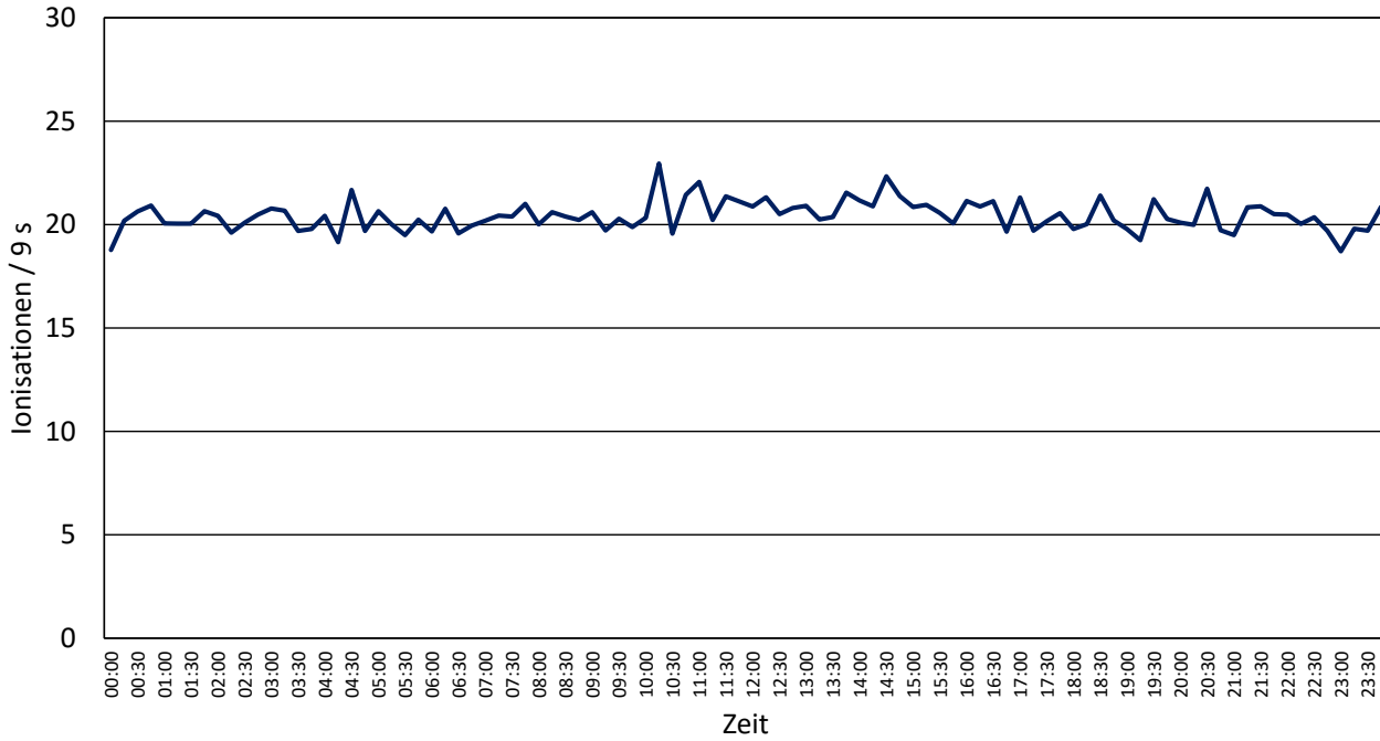
Anzahl Ionisationen
